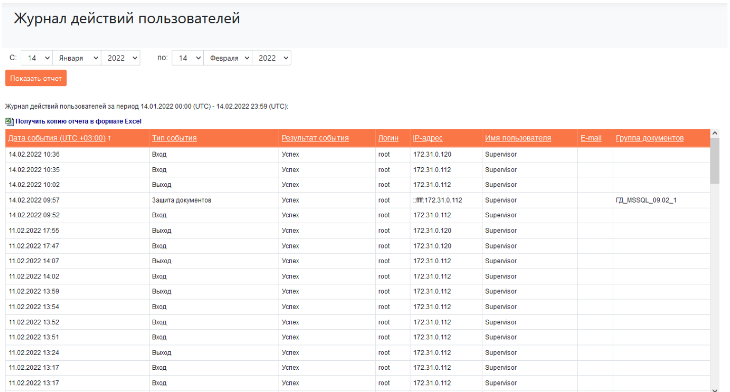
Рис. 18. Журнал действий пользователей. Подробная информация
